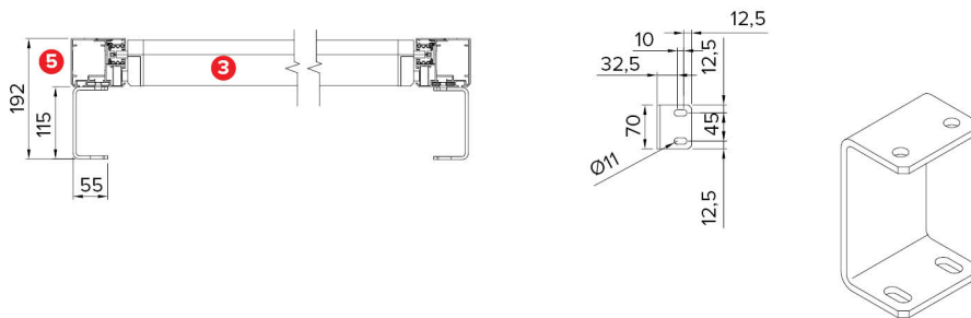
Dettaglio frangivento . Wind-break detail 088-930
